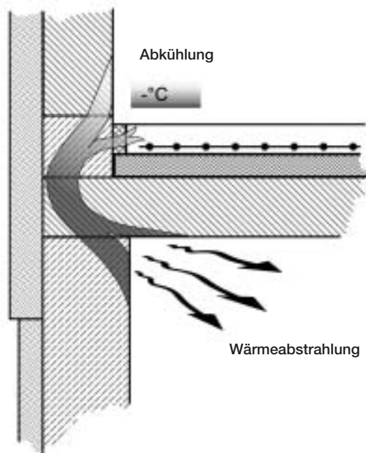
Abb. 33: Tiefgaragendecke mit Wärmefluss
